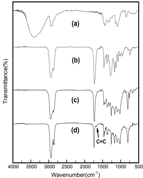
Figure 2. FT-IR spectra of (a) poly(vinyl alcohol); (b) PCALE3; (c) PCALE5; (d) PCALE10.
