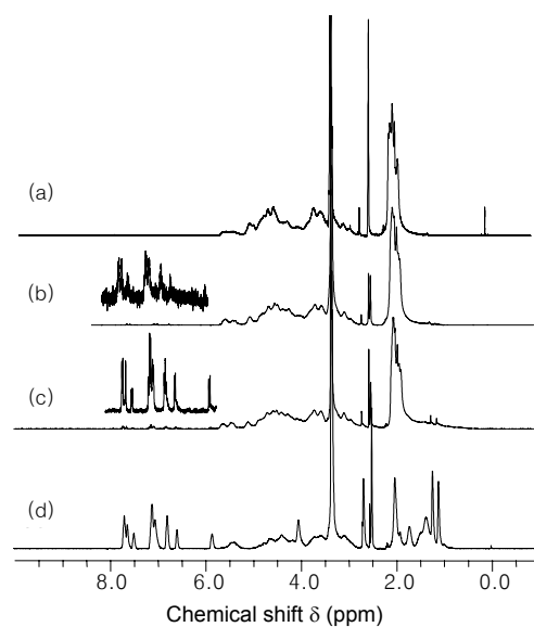
Figure 2. 1 H-NMR spectra of (a) CA, (b) CA-COSP1, (c) CA-COSP2, and (d) CA-COSP3 in DMSO- d 6 .
